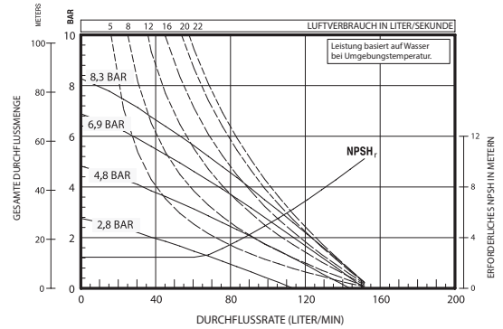
6661XX-XXX-C METALLISCHE 1"-MEMBRANPUMPE
