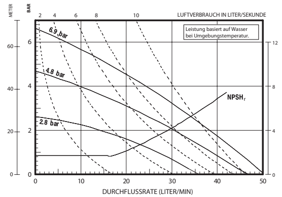
66605X-XXX NICHTMETALLISCHE 1/2"-MEMBRANPUMPE
